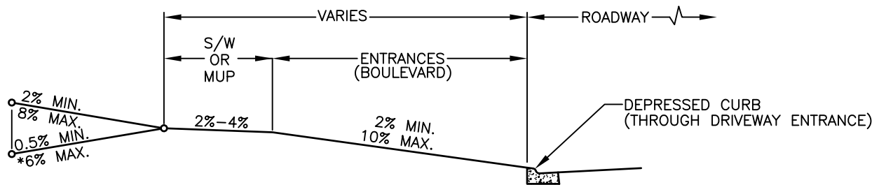
PROFILE DETAILS N.T.S.
